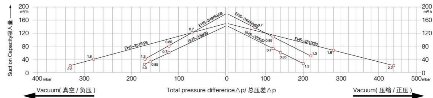
Vacuum Selection diagram 50 Hz--真空选型图表 50Hz
