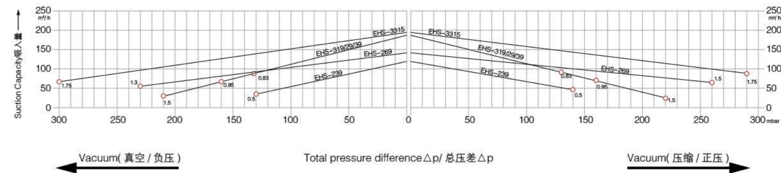
Vacuum Selection diagram 60 Hz--真空选型图表 60Hz
